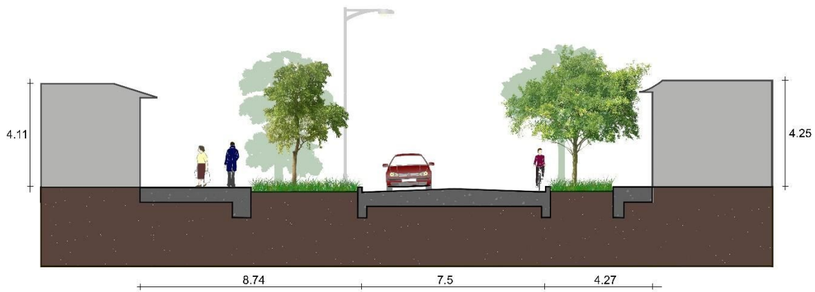
Perfil de calle San Francisco.
