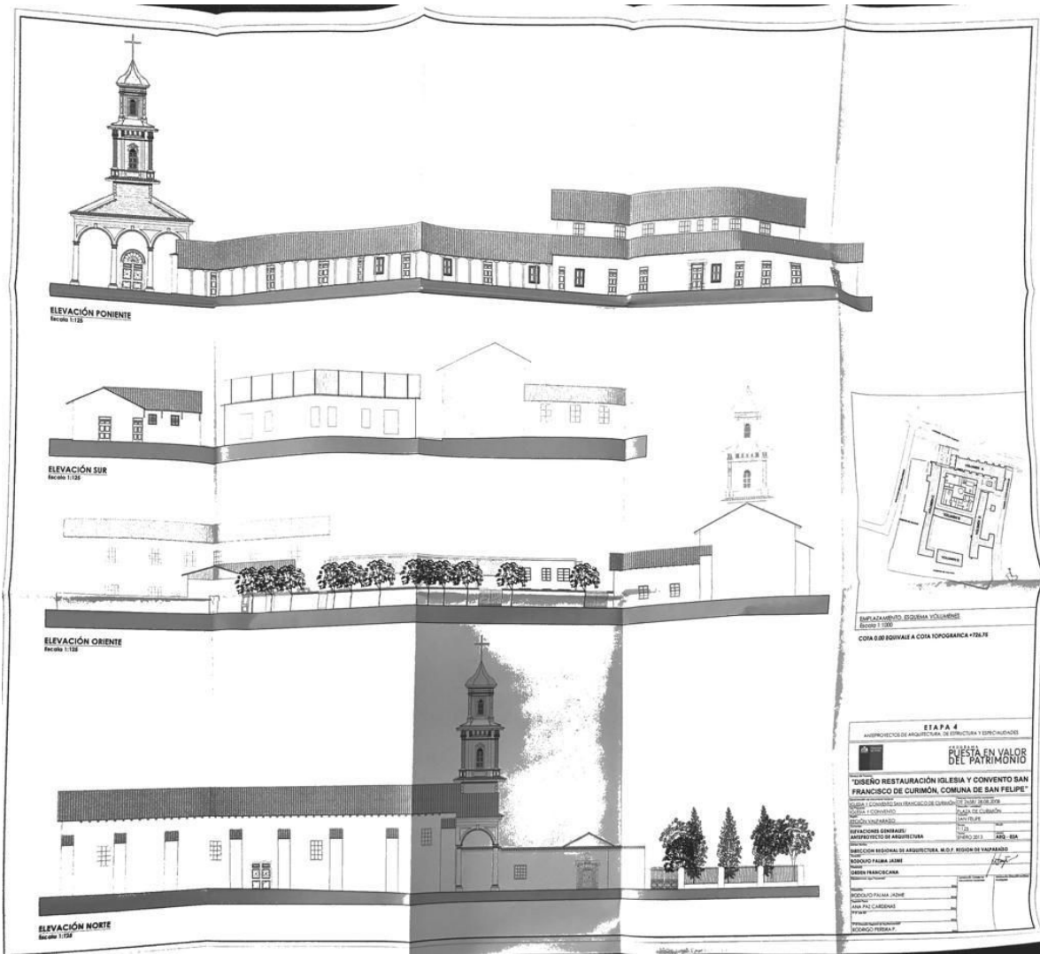
Elevaciones Iglesia y Convento San Francisco. Nacionales.
